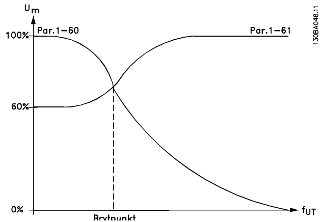
Bild 3.9 Lastkompensation för lågt varvtal
