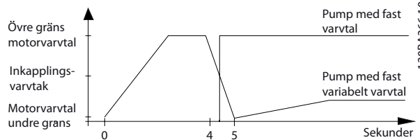
Bild 3.76 Inkopplingströskel
