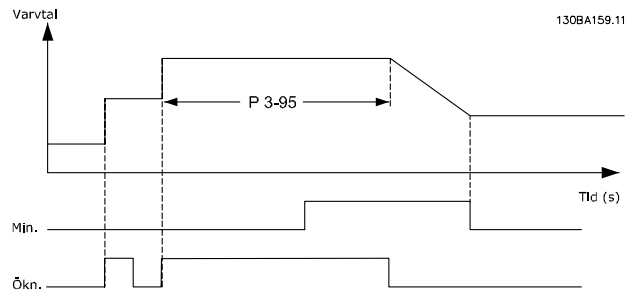
Bild 3.18 Rampfördröjning, fall 2
