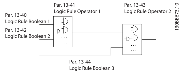
Bild 3.31 Logiska regler
