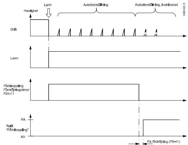
Bild 3.64 Förbikoppling
