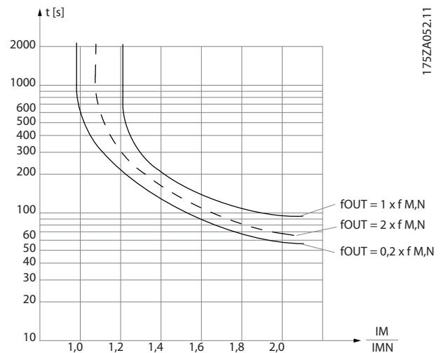
Bild 3.10 Termiskt motorskydd
