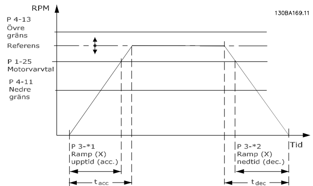
Bild 3.15 Ramp 1
