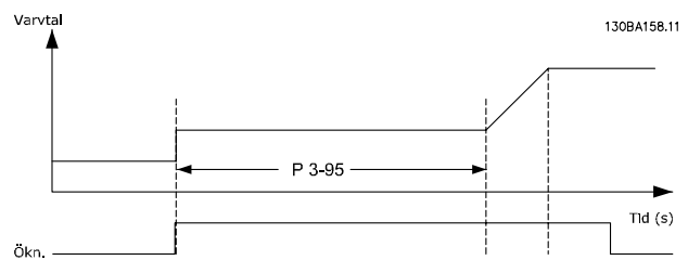
Bild 3.17 Rampfördröjning, fall 1
